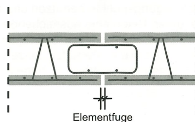
Horizontalschnitt Wand
